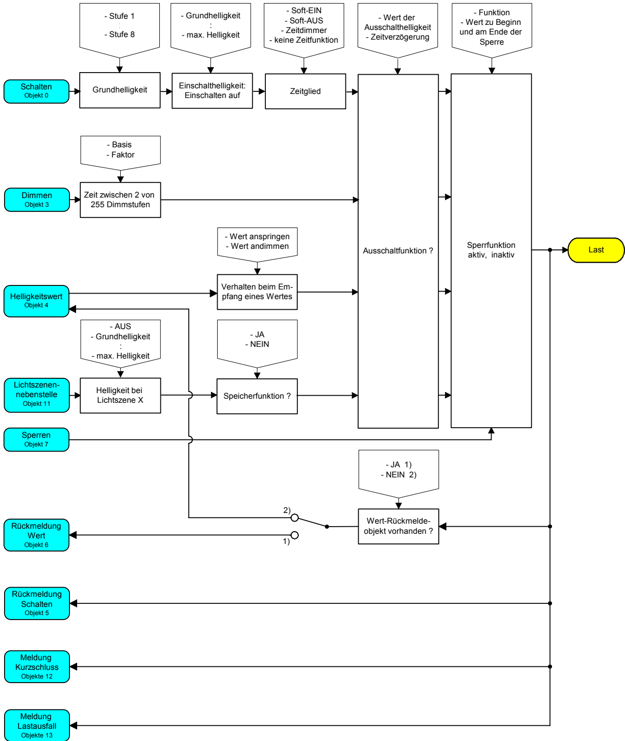
Funktionsschaltbild (für Dimmausgang)
